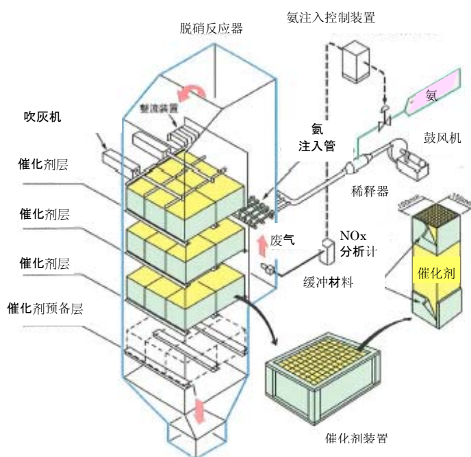
↑ 煤炭锅炉用脱硝系统例
