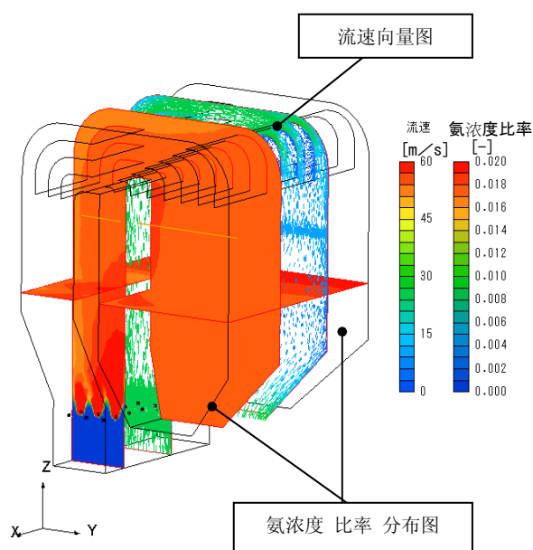
↑ 气体流程分析 (CFD)
