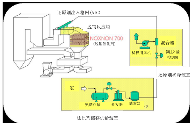
↑ 脱硝装置系统构成例：在氨（液氨）时
