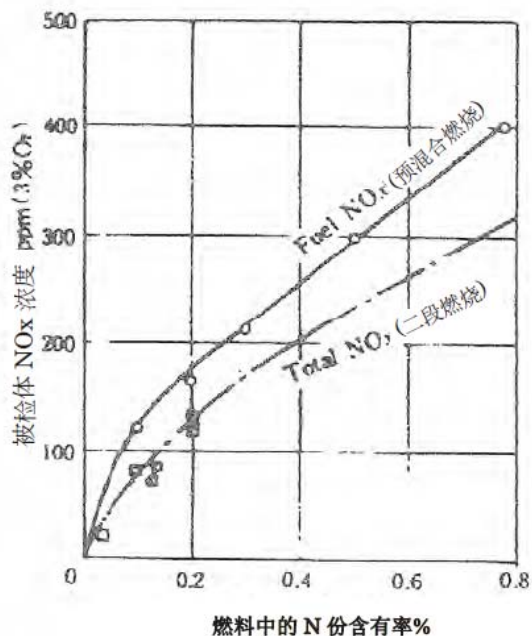
二段燃烧对降低 NO x 的效果
