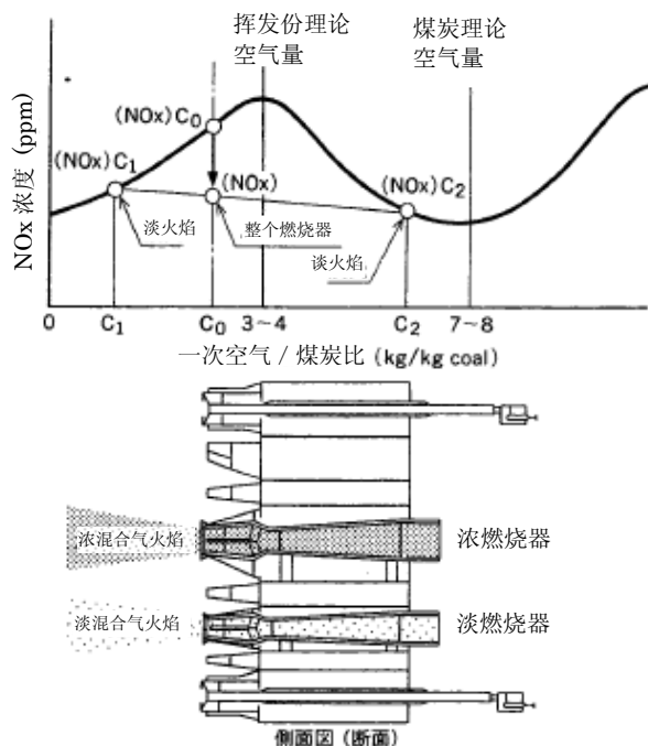
(a) 燃煤炭低 NO x 燃烧器
