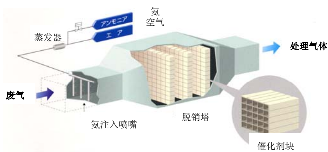
↑ 原理说明图
