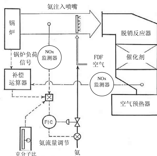
图 1 脱硝装置的运转控制图
