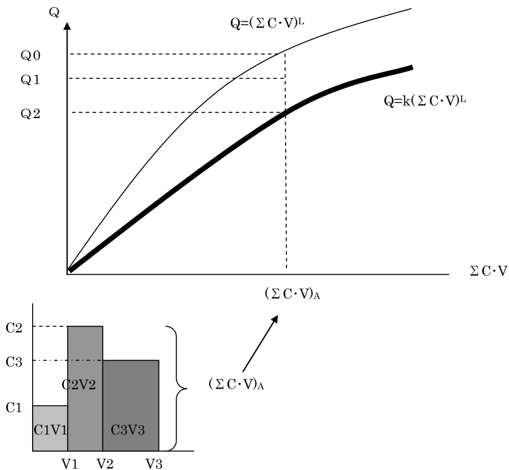
図 4.1-2 基礎排出量算定方式
