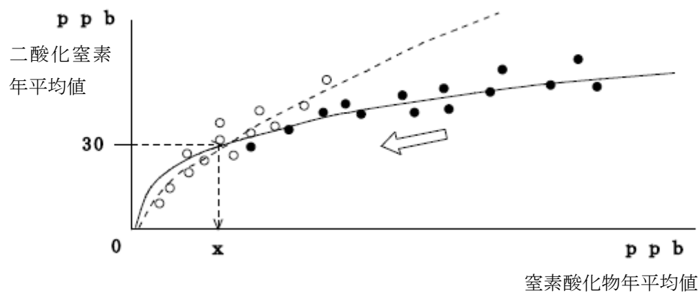
図 5.2-1 二酸化窒素濃度と窒素酸化物濃度との関係
