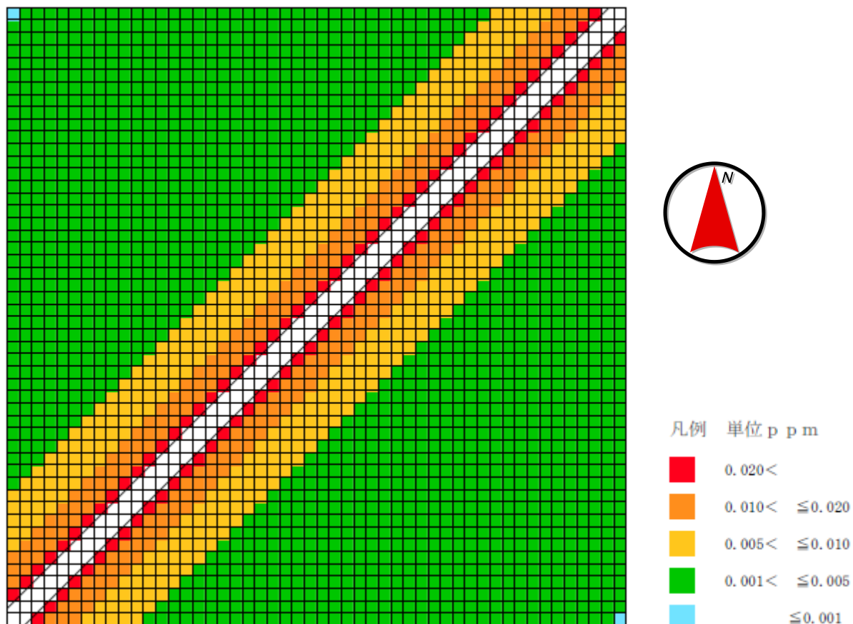
図 6.2-1 道路沿道の窒素酸化物濃度分布 (低中層建物が散在している場合) (図中の白い部分は道路を表す。1 格子は 10m×10m。縮尺 1/5000。)
