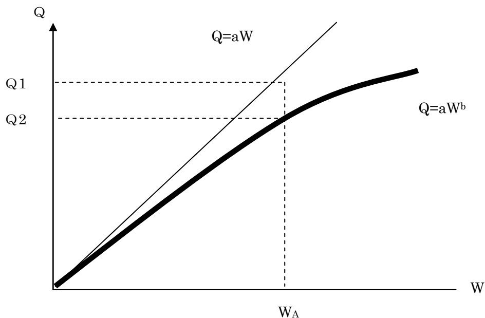
図 4.1-1 原燃料使用量方式
