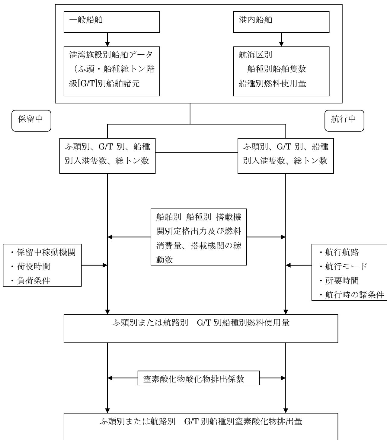
図 2.5-1 船舶からの窒素酸化物排出量の算定フロー
