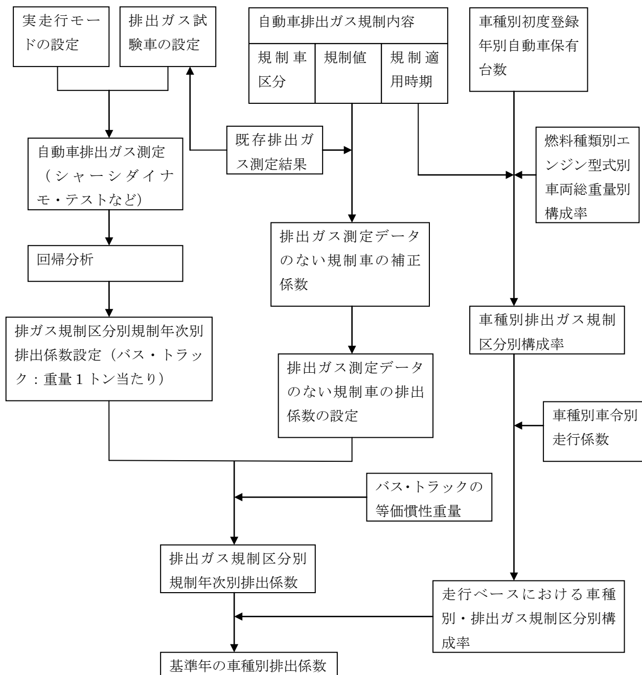
図 2.4-2 窒素酸化物排出係数の設定作業フロー
