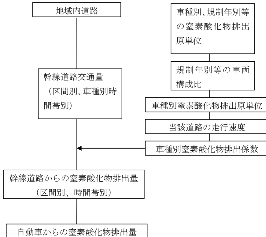
図 2.4-1 幹線道路を走行する自動車からの窒素酸化物排出量算定フロー
