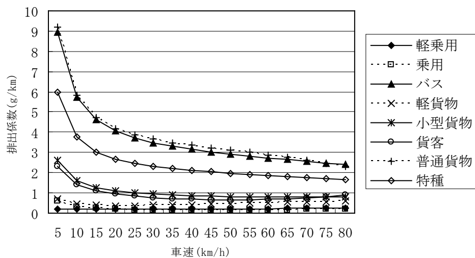
図 2.4-3 車種別の窒素酸化物排出係数 ( E F_i ) の例
