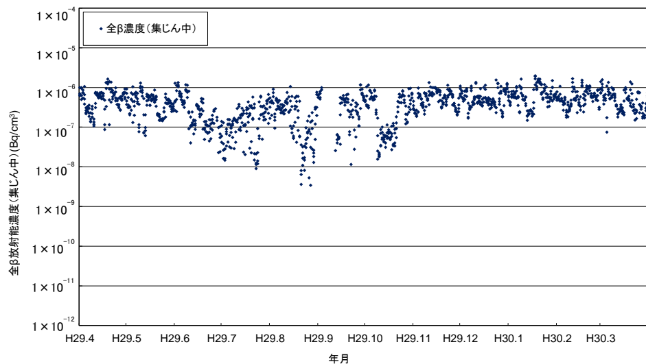
辺戸岬測定所における大気浮遊jinの全β放射能濃度(集jin中)の経時変化
