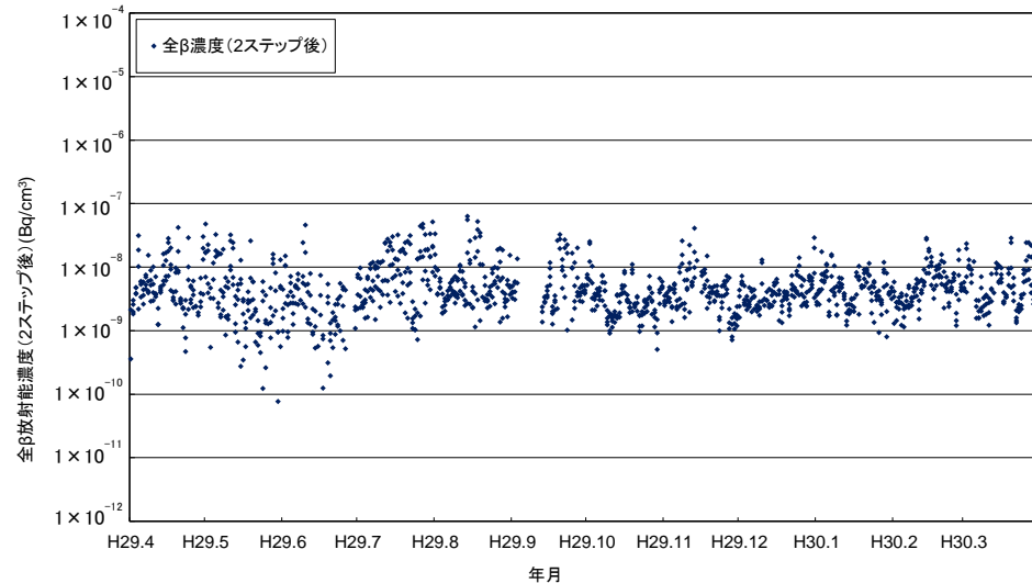
辺戸岬測定所における大気浮遊jinの全β放射能濃度(2ステップ後)の経時変化
