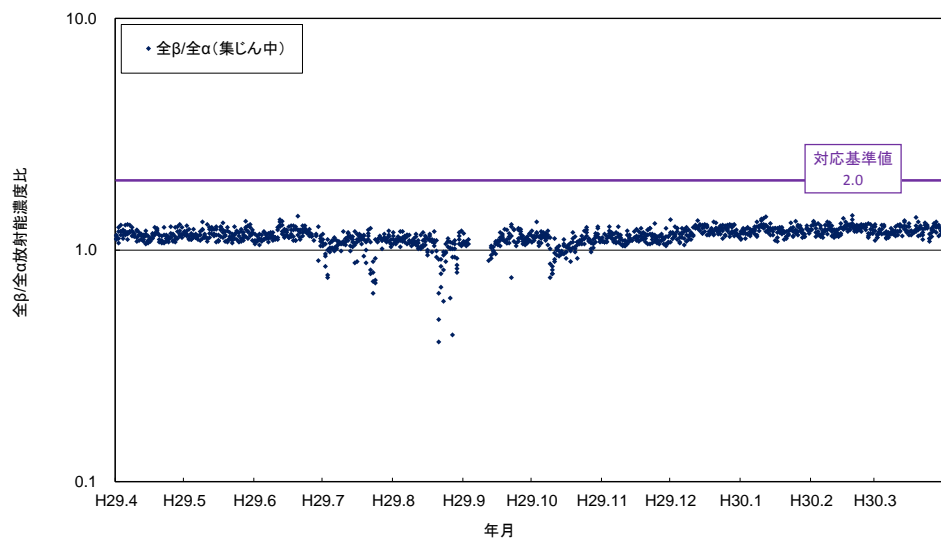
辺戸岬測定所における大気浮遊jinの全β/全α放射能濃度比(集jin中)の経時変化
