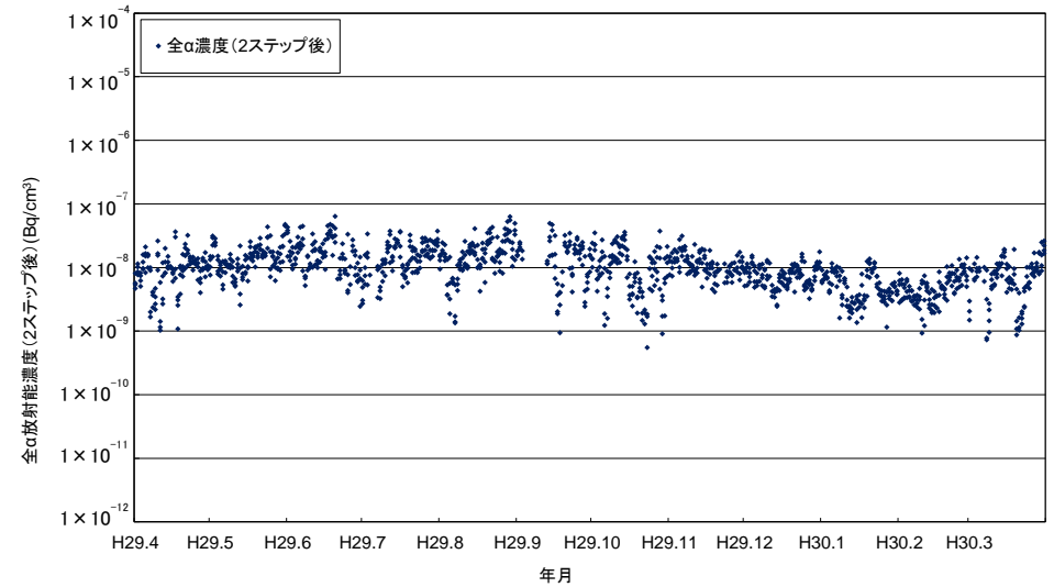
橋原測定所における大気浮遊じん全α放射能濃度(2ステップ後)の経時変化
