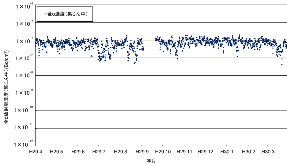
対馬測定所における大気浮遊じん的全α放射能濃度(集じん中)の経時変化
