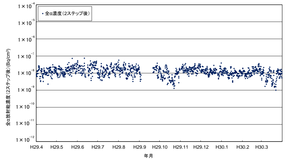
対馬測定所における大気浮遊じん的全α放射能濃度(2ステップ後)の経時変化
