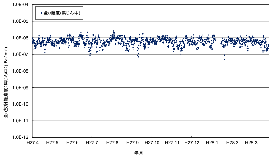
付図4-16 越前岬測定所における大気浮遊じんの大α放射能濃度（集じん中）の経時変化
