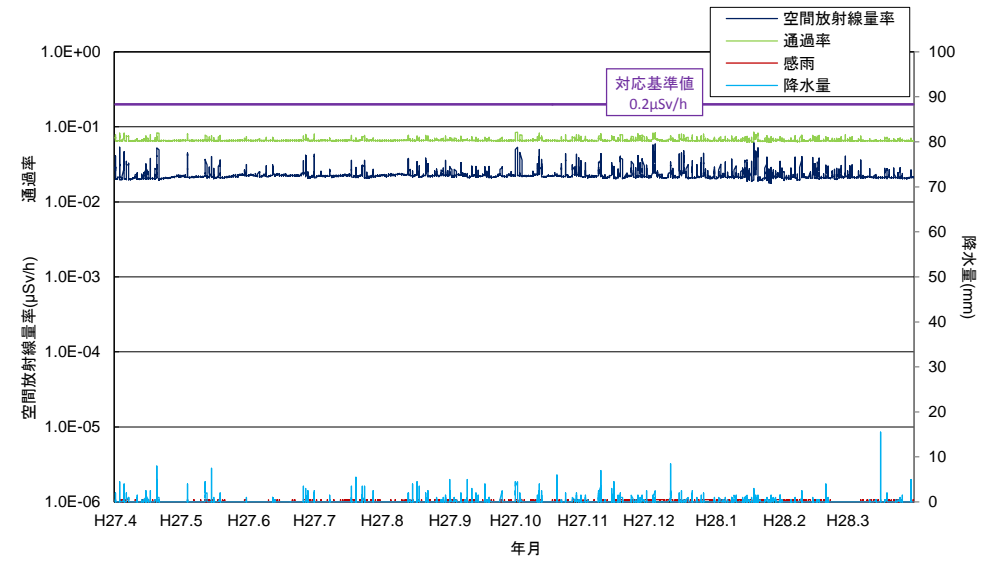
付図3-3 佐渡関岬測定所における空間放射線量率及び降水量との関係
