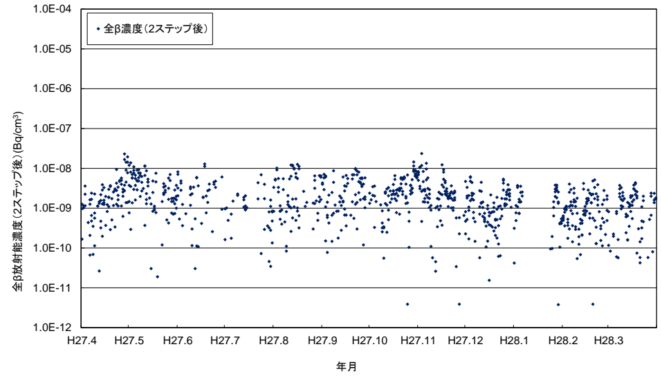
付図4-4 利尻測定所における大気浮遊じんの全β放射能濃度(2ステップ後)の経時変化
