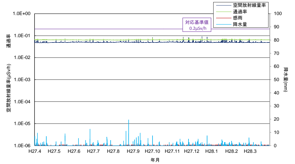
付図3-5 隠岐測定所における空間放射線量率及び降水量との関係
