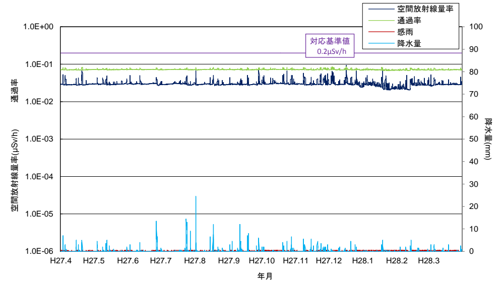
付図3-2 竜飛岬測定所における空間放射線量率及び降水量との関係
