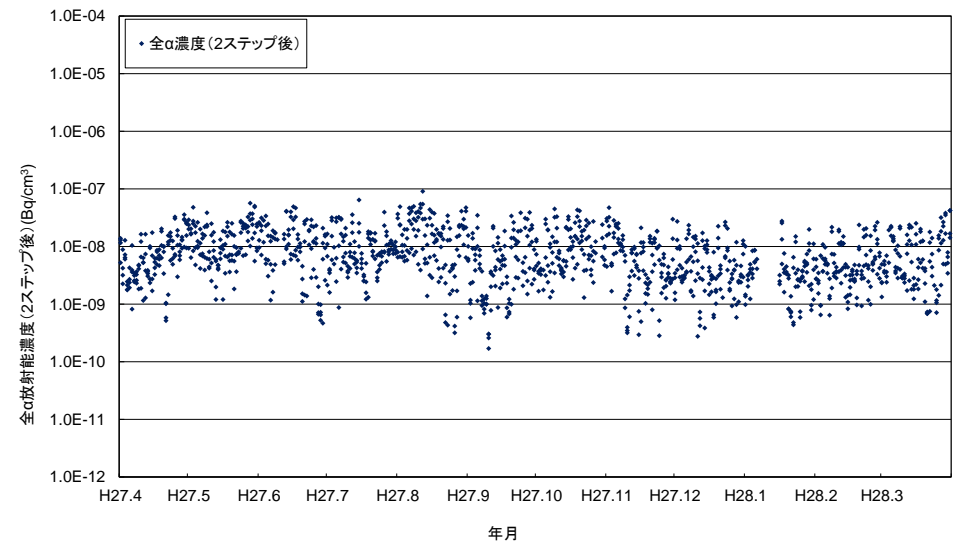
付図4-22 隠岐測定所における大気浮遊じんの全α放射能濃度（2ステップ後）の経時変化
