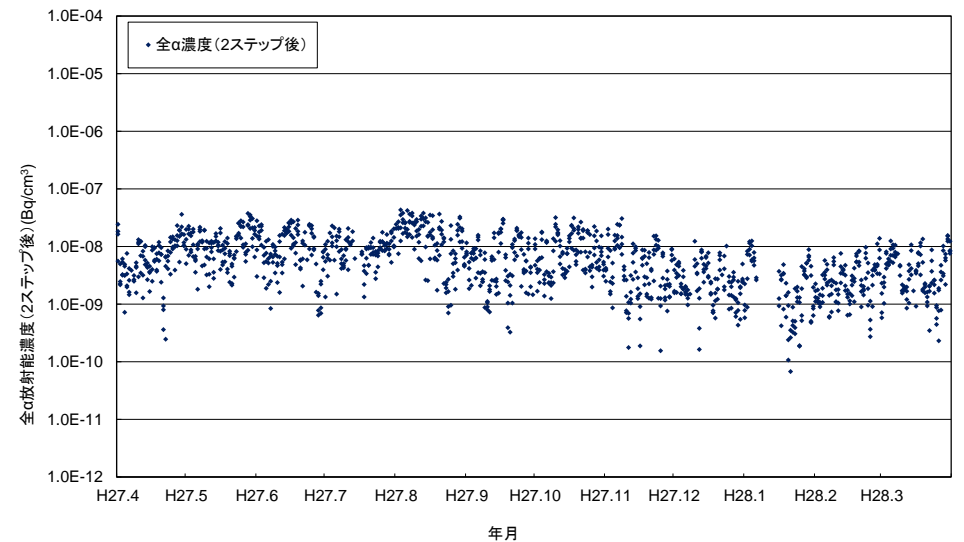
付図4-17 越前岬測定所における大気浮遊じんの大α放射能濃度（2ステップ後）の経時変化
