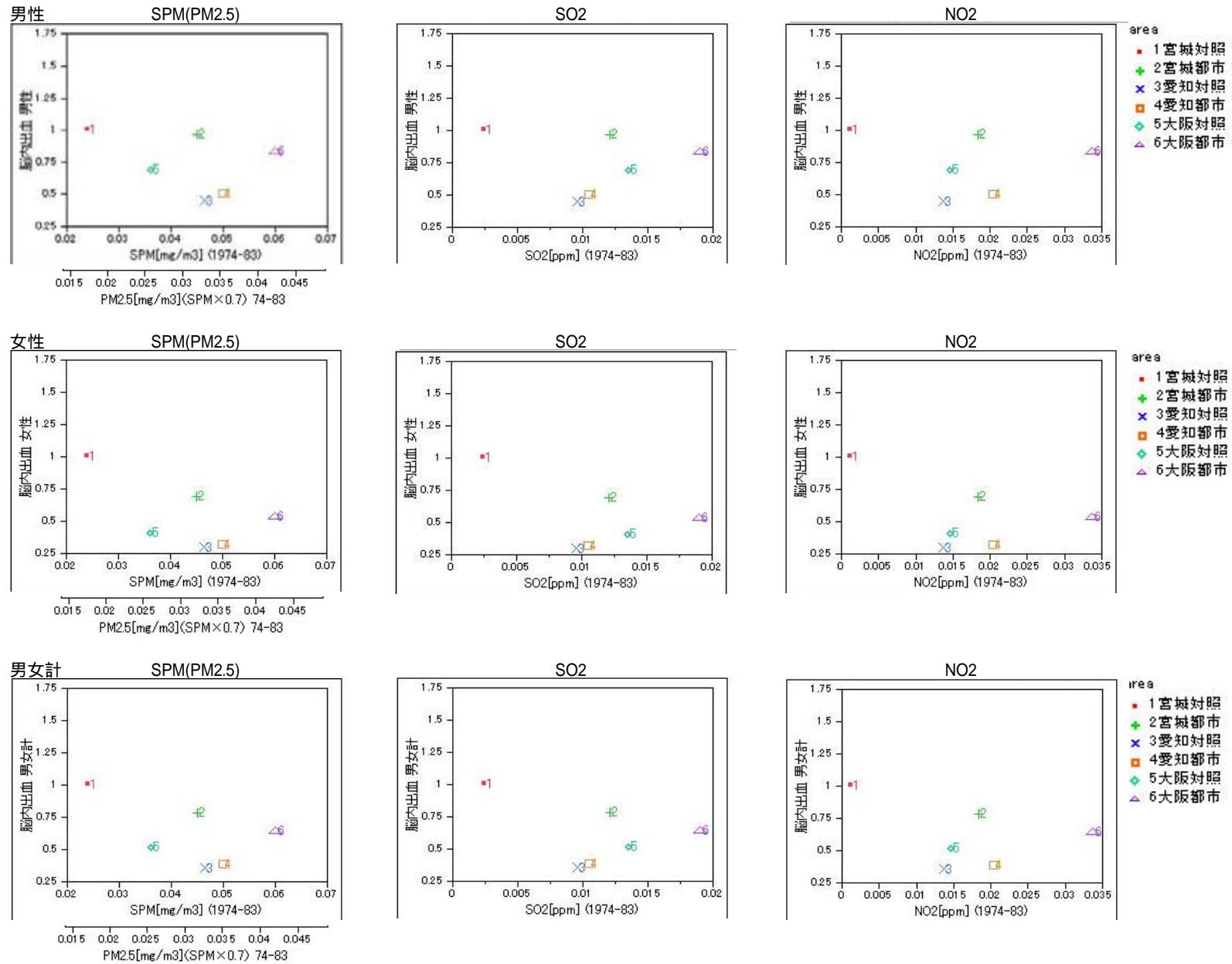
図5-1-11.大気と相対リスクのプロット_脳内出血_10年追跡
