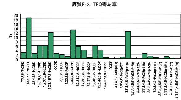
参考図 2 - 10 共通試料 F-3 の異性体パターン
