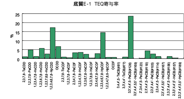
参考図2 - 1 共通試料 E-1 の異性体パターン
