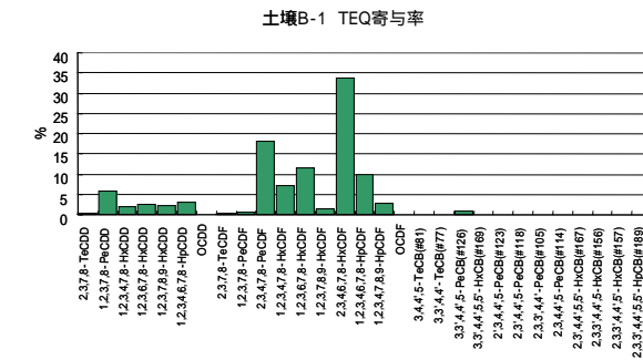
参考図 1 - 8 共通試料 B-1 の異性体パターン
