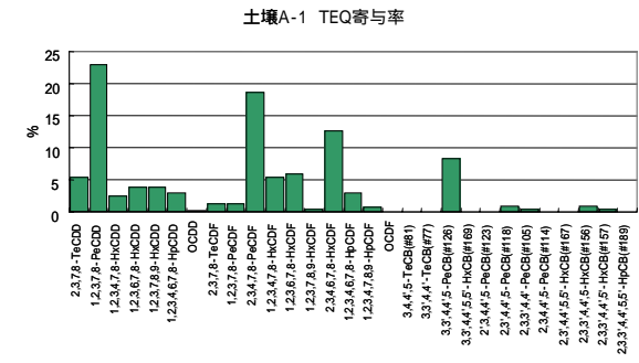
参考図 1 - 1 共通試料 A-1の異性体パターン
