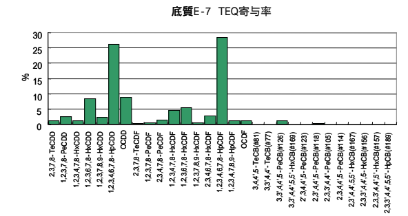
参考図 2 - 7 共通試料 E-7 の異性体パターン
