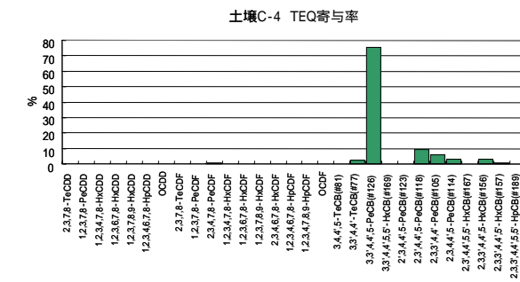
参考図 1 - 13 共通試料 C-2 の異性体パターン 参考図 1 - 14 共通試料 C-3 の異性体パターン 参考図 1 - 15 共通試料 C-4 の異性体パターン
