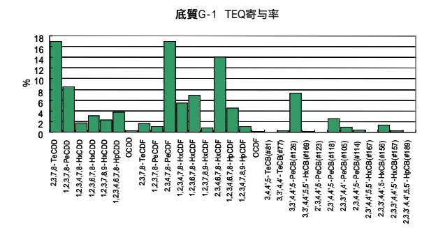
参考図 2 - 11 共通試料 G-1 の異性体パターン
