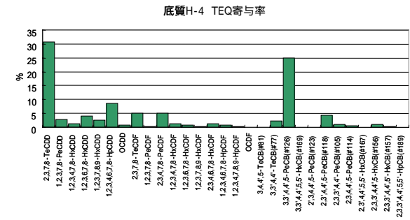
参考図 2 - 18 共通試料 H-4 の異性体パターン
