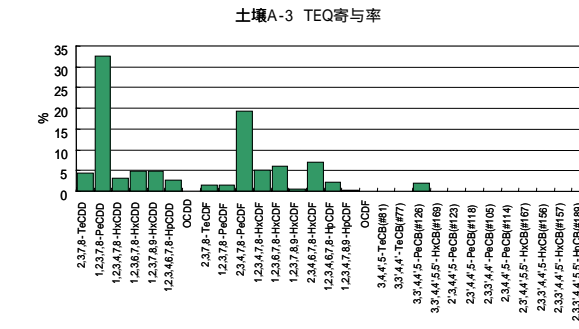
参考図 1 - 3 共通試料 A-3の異性体パターン
