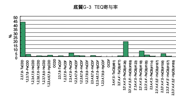
参考図 2 - 1 3 共通試料 G-3 の異性体パターン
