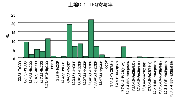
参考図 1 - 16 共通試料 D-1 の異性体パターン 参考図 1 - 17 共通試料 D-2 の異性体パターン 参考図 1 - 18 共通試料 D-3 の異性体パターン
