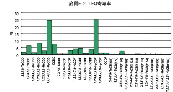
参考図2 - 2 共通試料 E-2 の異性体パターン
