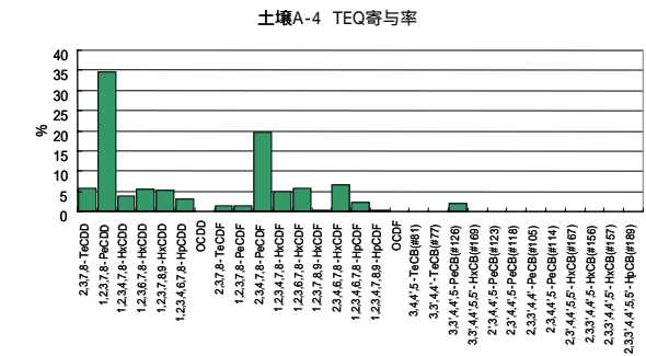
参考図 1 - 4 共通試料 A-4の異性体パターン
