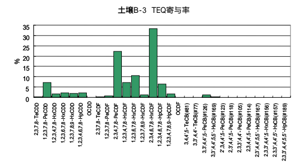
参考図1-10 共通試料 B-3 の異性体パターン 参考図1-11 共通試料 B-4 の異性体パターン 参考図1-12 共通試料 C-1 の異性体パターン
