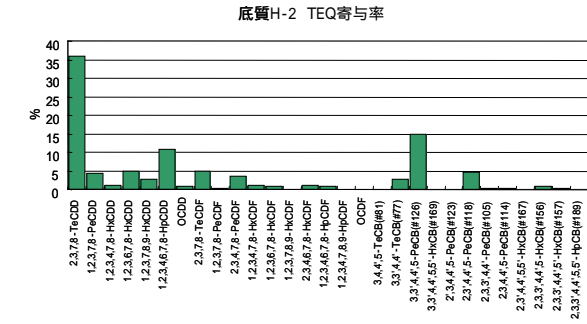
参考図 2 - 16 共通試料 H-2 の異性体パターン
