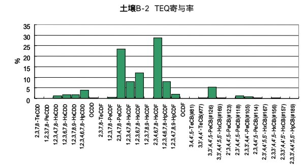
参考図 1 - 9 共通試料 B-2 の異性体パターン
