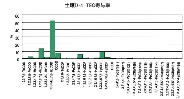
参考図1 - 19 共通試料 D-4 の異性体パターン
