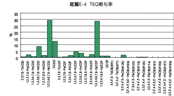
参考図 2 - 4 共通試料 E-4 の異性体パターン
