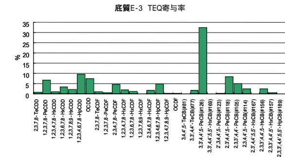
参考図 2 - 3 共通試料 E-3 の異性体パターン
