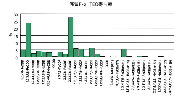
参考図 2 - 9 共通試料 F-2 の異性体パターン
