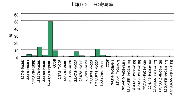
参考図 1 - 16 共通試料 D-1 の異性体パターン 参考図 1 - 17 共通試料 D-2 の異性体パターン 参考図 1 - 18 共通試料 D-3 の異性体パターン
