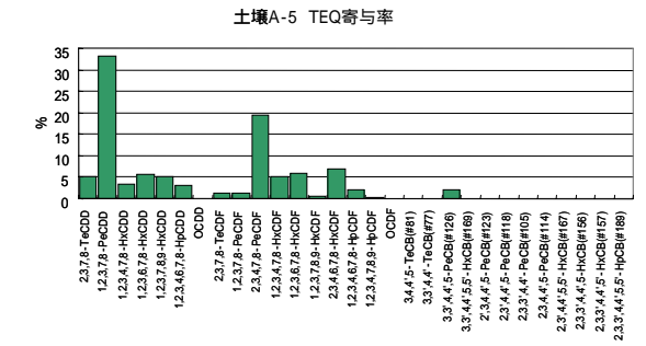
参考図 1 - 5 共通試料 A-5の異性体パターン
