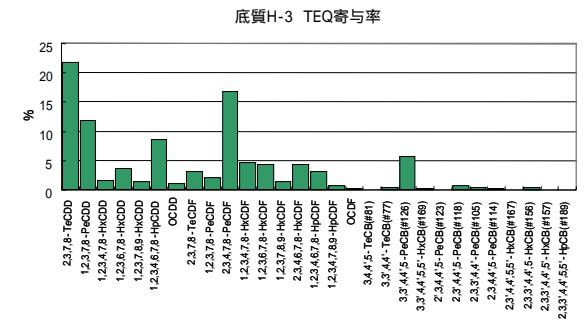
参考図 2 - 17 共通試料 H-3 の異性体パターン
