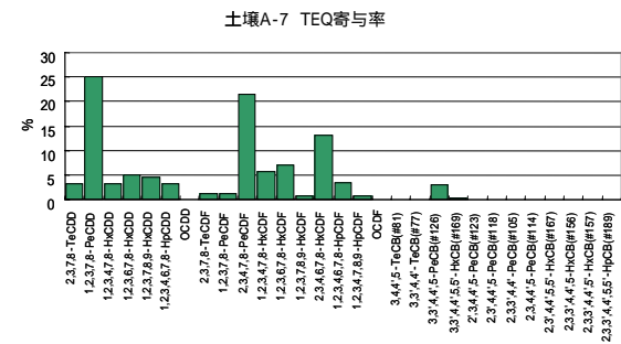
参考図 1 - 7 共通試料 A-7 の異性体パターン
