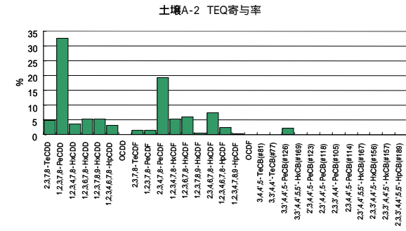
参考図 1 - 2 共通試料 A-2の異性体パターン
