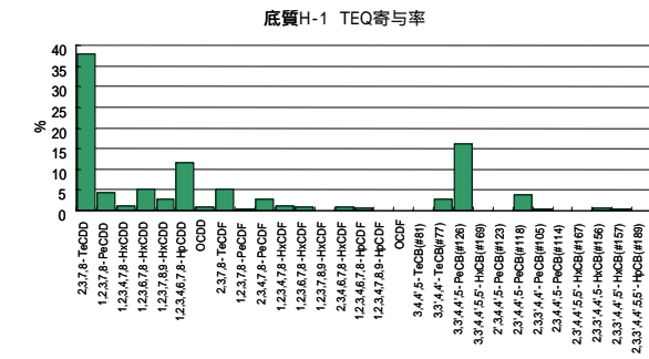
参考図 2 - 15 共通試料 H-1 の異性体パターン
