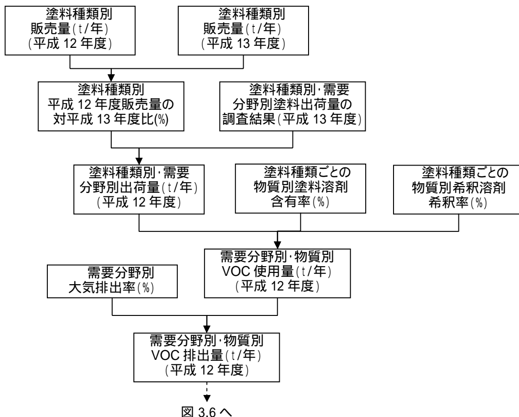
図 3.5 塗料の使用に係る業種別・物質別 VOC 排出量の推計フロー(平成 12 年度分のみ)
