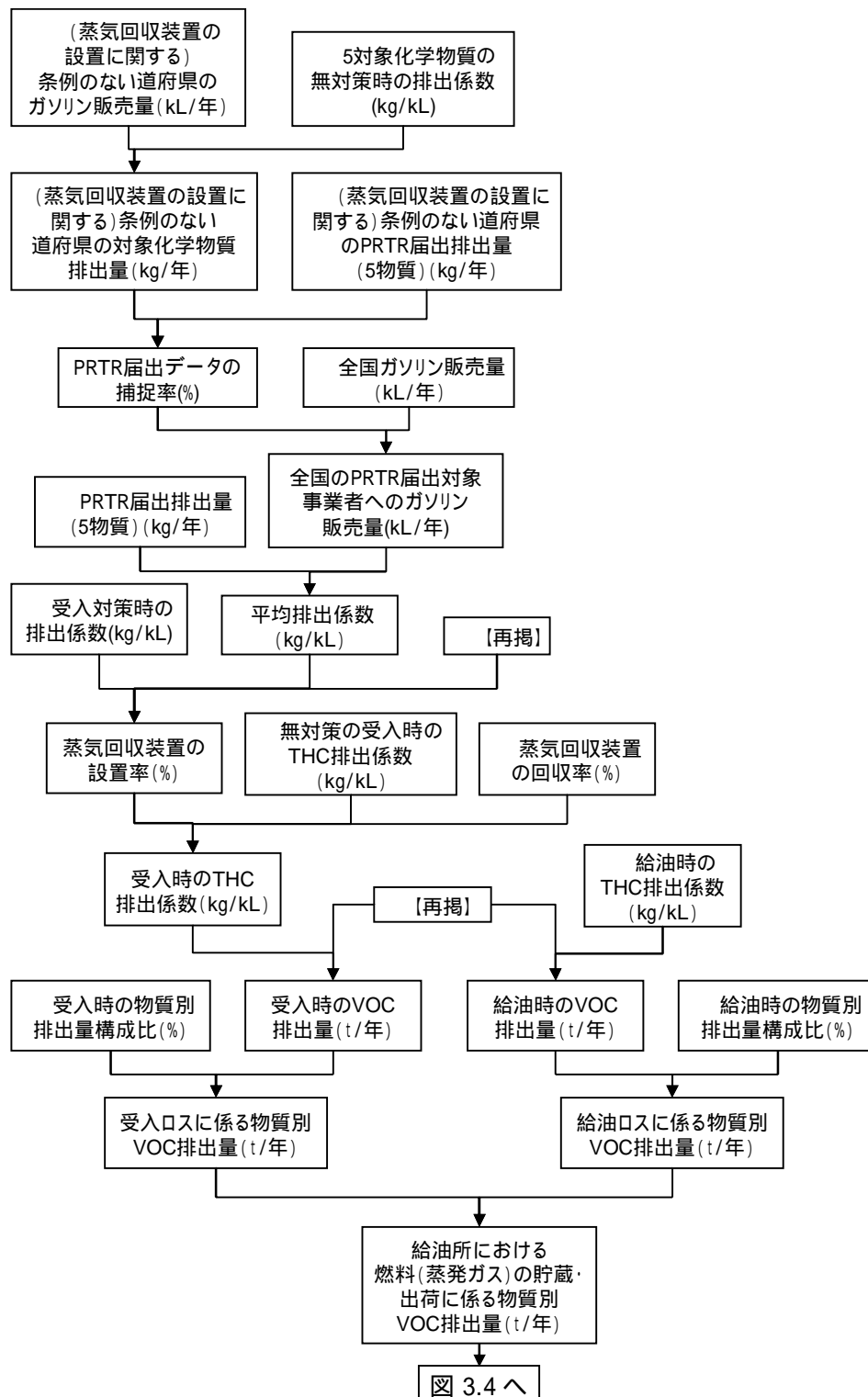
図 3.3 給油所における燃料(蒸発ガス)の貯蔵・出荷に係る物質別 VOC 排出量の推計フロー
