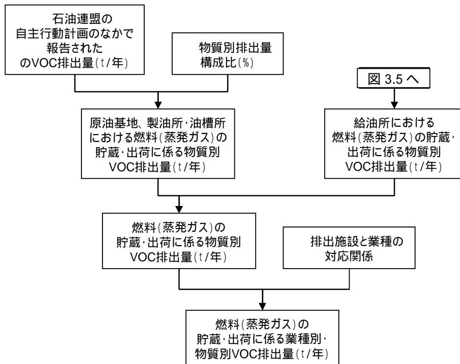
図 3.4 燃料(蒸発ガス)に係る貯蔵・出荷に係る業種別・物質別 VOC 排出量の推計フロー
