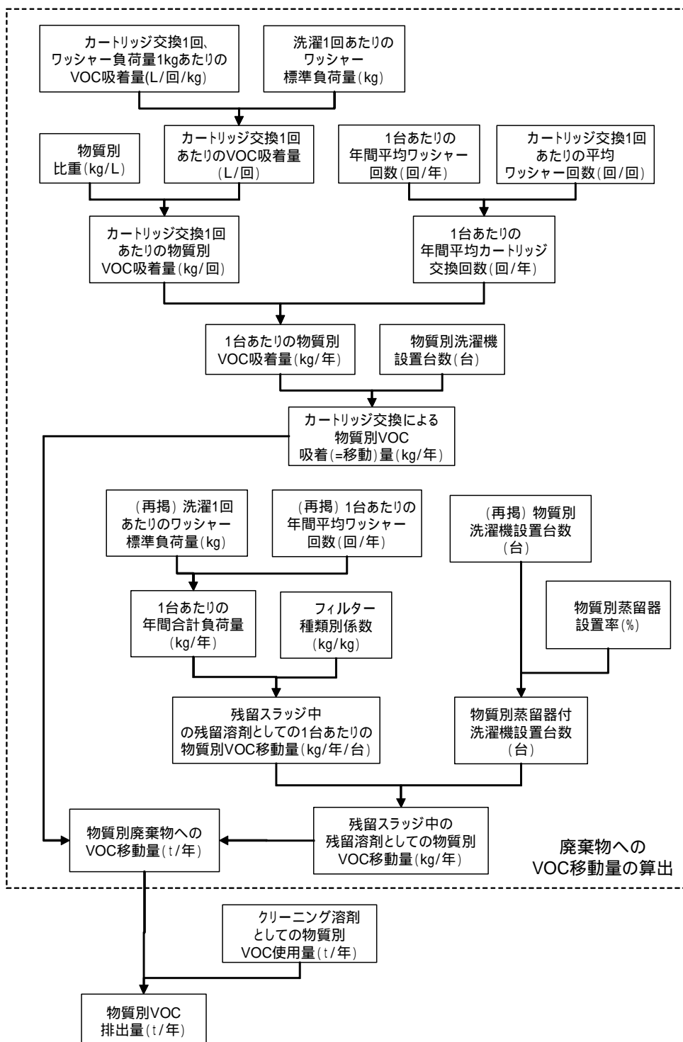
図 3.12 ドライクリーニング溶剤の使用に係る業種別・物質別 VOC 排出量の推計フロー
