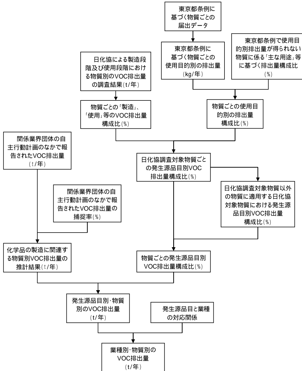
図 3.2 化学品の製造に関連する発生源品目別・物質別 VOC 排出量の推計フロー
