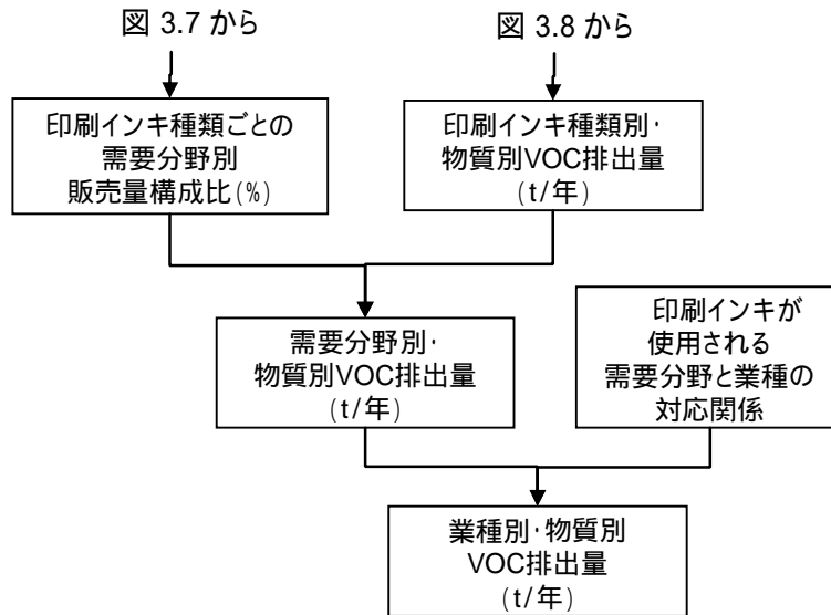
図 3.9 印刷インキの使用に係る業種別・物質別 VOC 排出量の推計フロー
