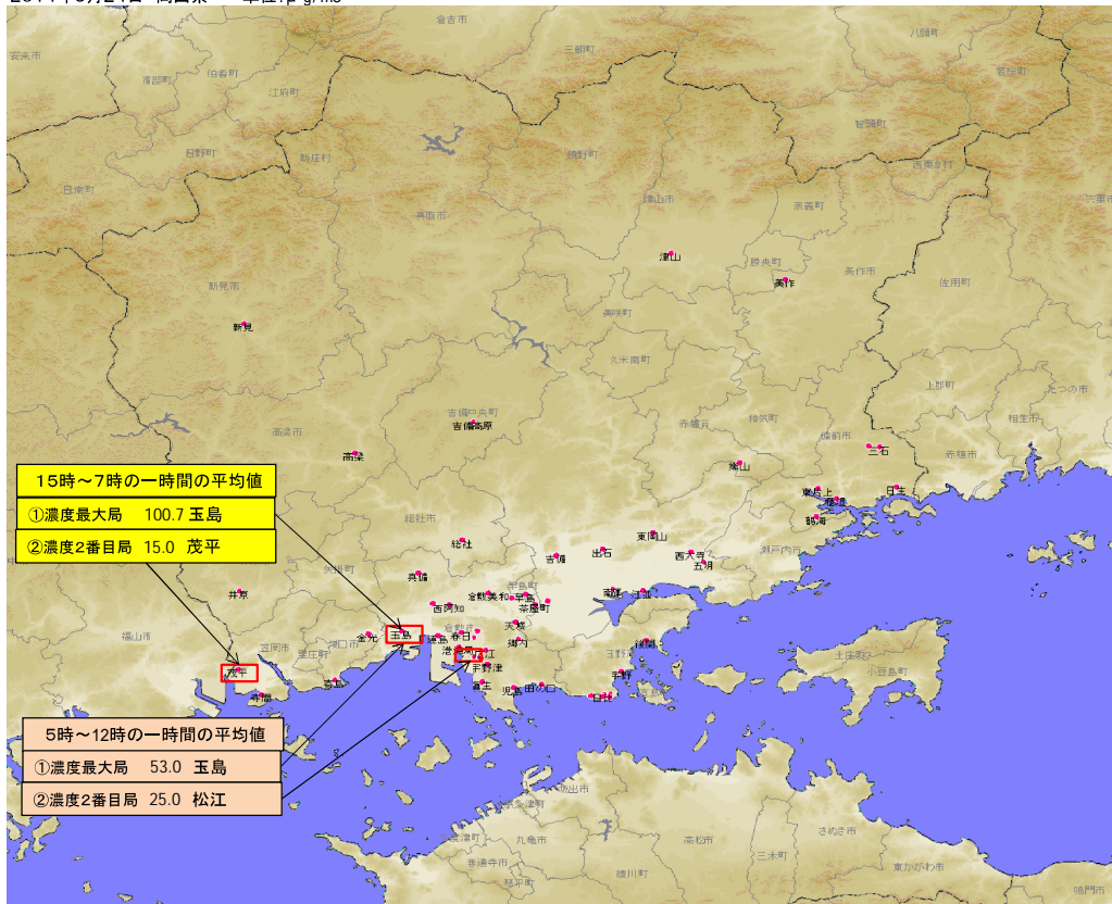
2014年5月24日 岡山県 単位: \mu\text{g}/\text{m}^3
