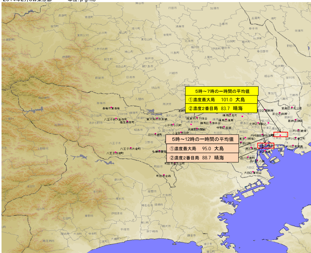
2014年2月3日東京都 単位: \mu\text{g}/\text{m}^3
