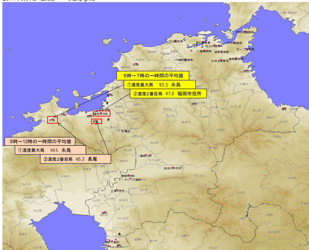
2014年6月1日 福岡県 単位: \mu\text{g}/\text{m}^3
