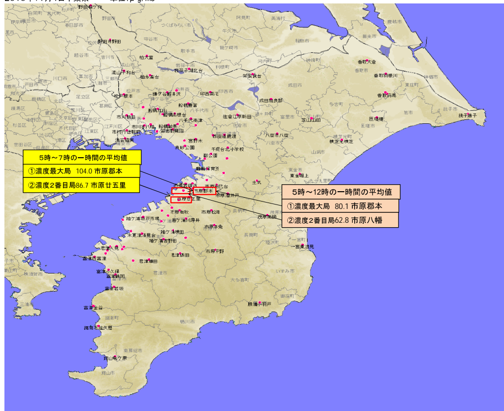
2013年11月4日千葉県 単位: \mu\text{g}/\text{m}^3
