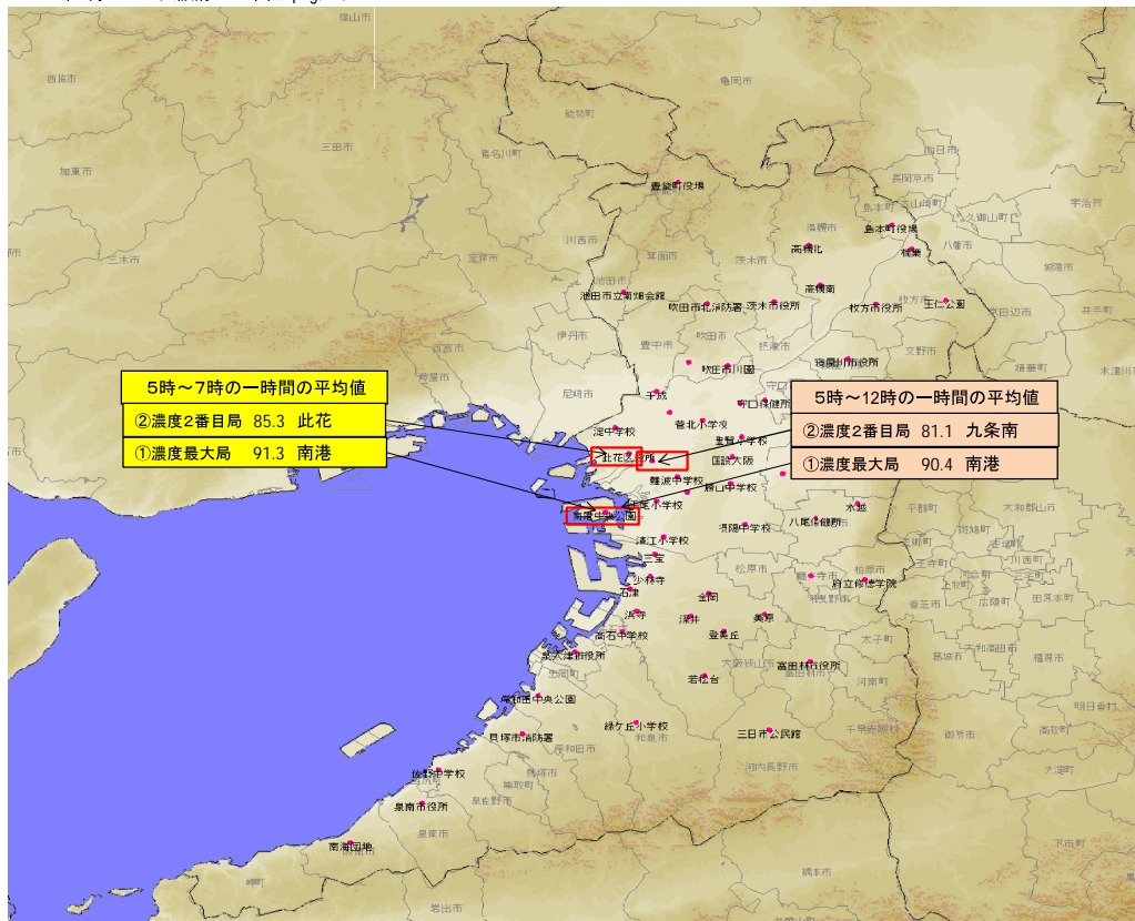
2014年2月26日 大阪府 単位: \mu\text{g}/\text{m}^3
