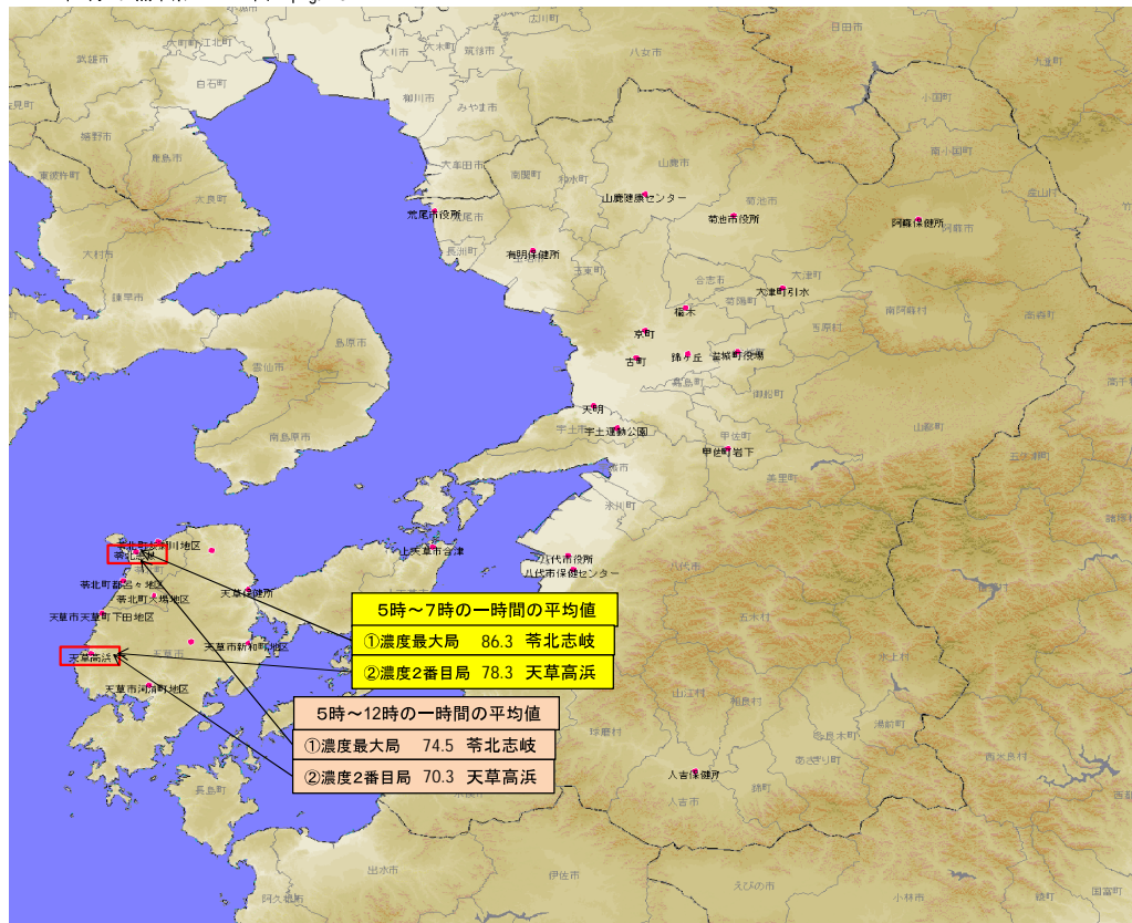
2014年2月3日熊本県 単位: \mu\text{g}/\text{m}^3
