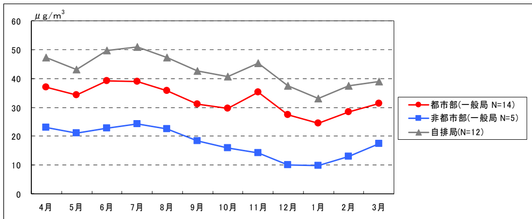
図1.2.3 SPM(β線)質量濃度の月変動(平成13~17年度の平均値) 【差し替え予定】 (1)
