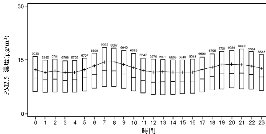
図 3.1.1.4 全米における PM 2.5 平均濃度の時間値（日内）変動。 四分位範囲、中央値、平均値(+)で示す。箱ひげ図上の数値は 1999 年の観測回数を表す。 典拠： Fitz-Simons ら (2000))
