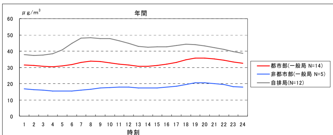
図1.2.5 SPM(β線)質量濃度の時間変動(平成13~17年度の平均値) 【差し替え予定】 (1)
