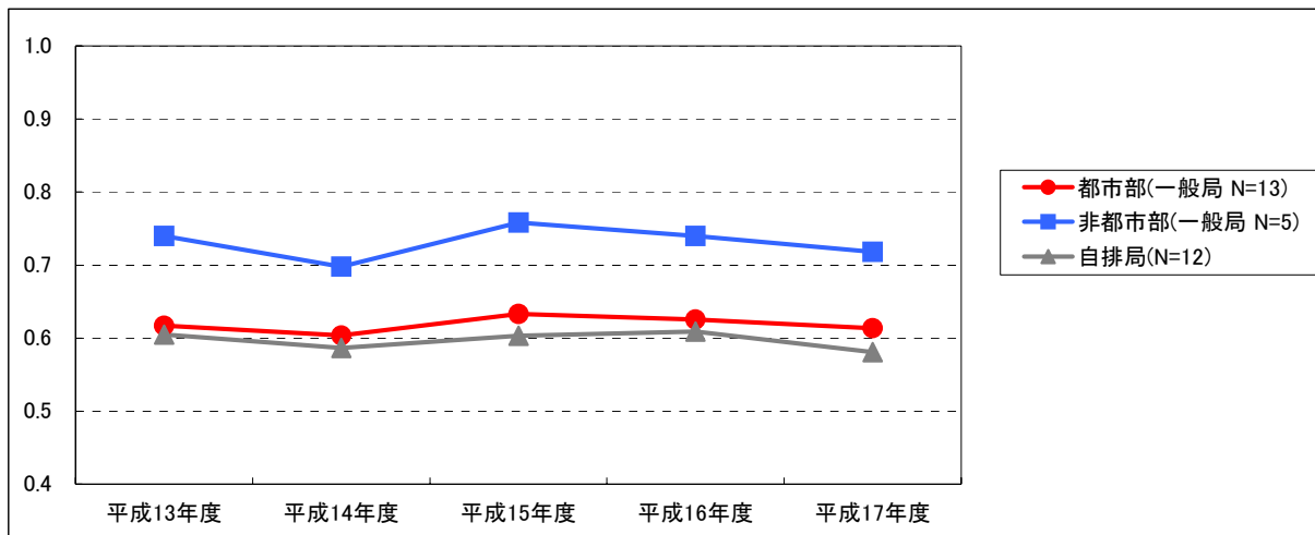
図1.2.7 PM 2.5 (TEOM)/SPM (β線) 比の年変動【差し替え予定】
