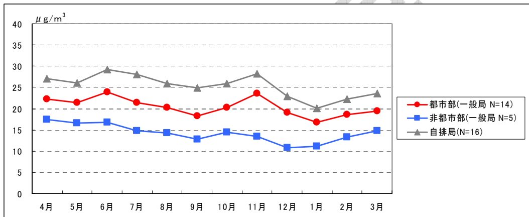
図1.2.4 PM 2.5 (TEOM)質量濃度の月変動(平成13~18年度の平均値) (1)
