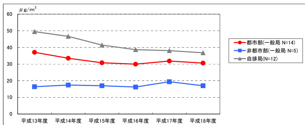
図1.2.1 SPM( \beta 線)質量濃度の年変動(1)
