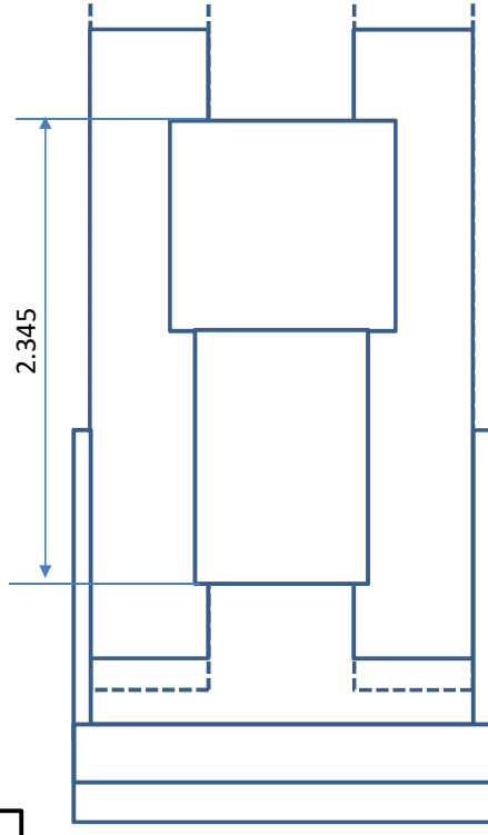
平面図
